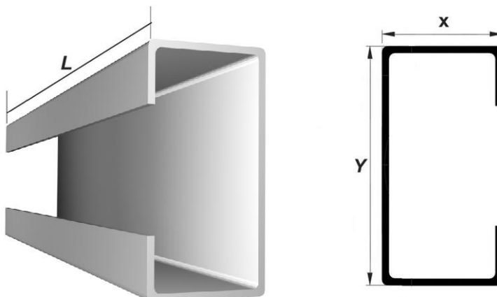
Figura 1 - Canaleta metálica
